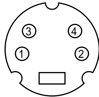
MINI DIN 4P MALE (TOP VIEW)
