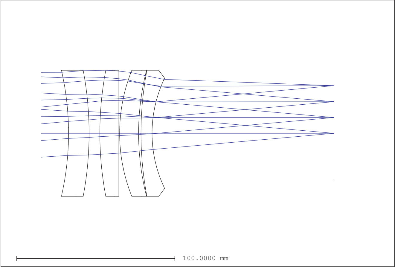
645レデューサー の断面図
