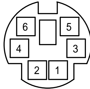
MINI DIN 6P FEMALE (TOP VIEW)
